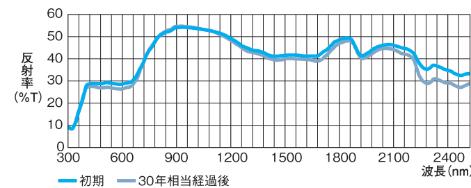
■耐候性試験分光光度計反射率測定データグラフ(グラッサ・クールシルバー)
